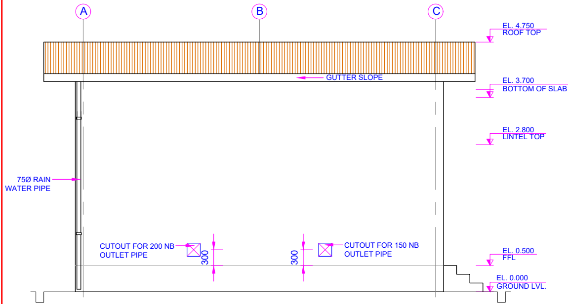
ELEVATION-A
